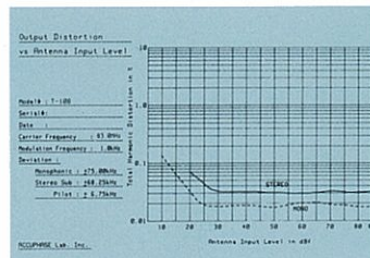
●入力信号レベル/全高調波ひずみ率特性
