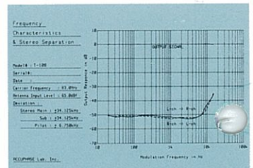
●周波数特性及びステレオ・セパレーション特性
